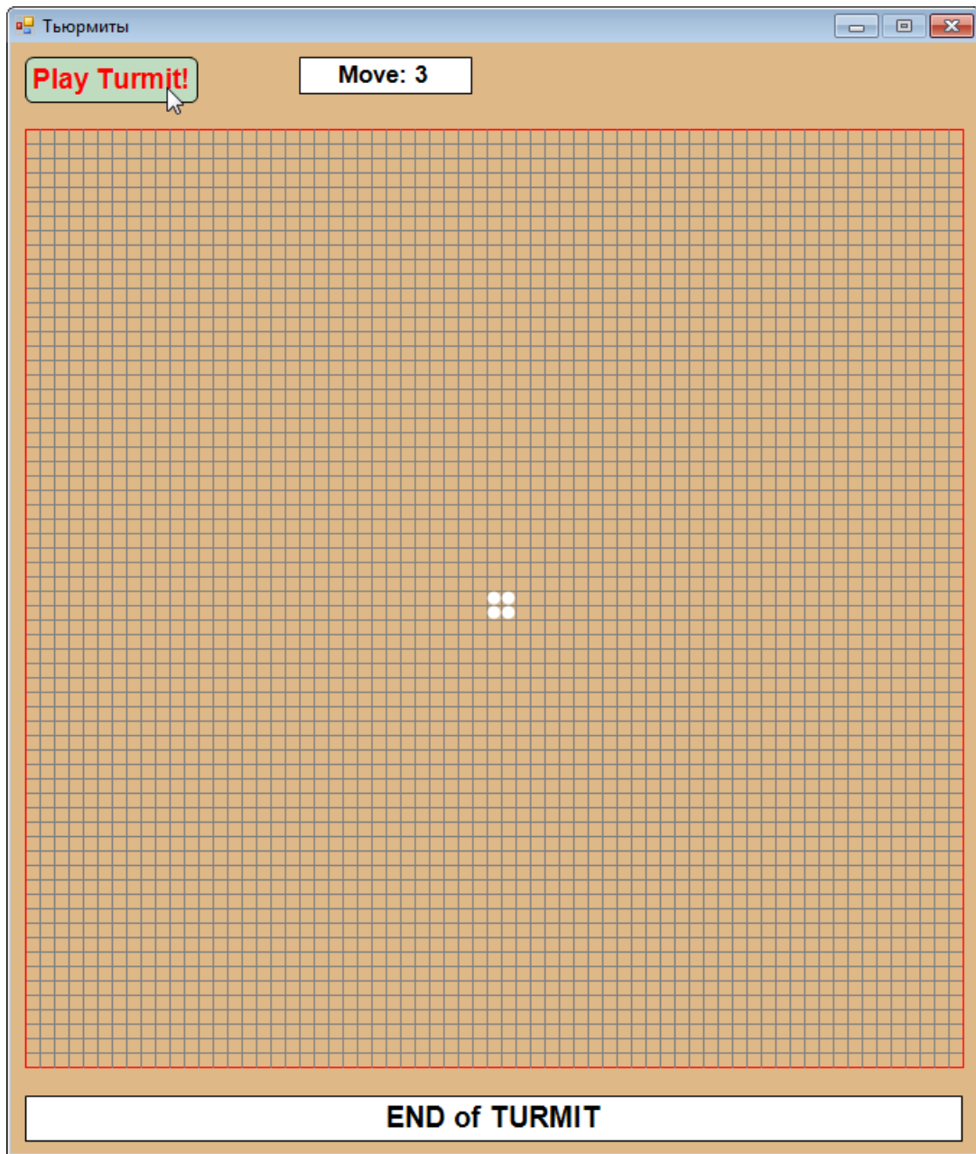
Рис. 24.18. Тьюрмит «оквадратился»
