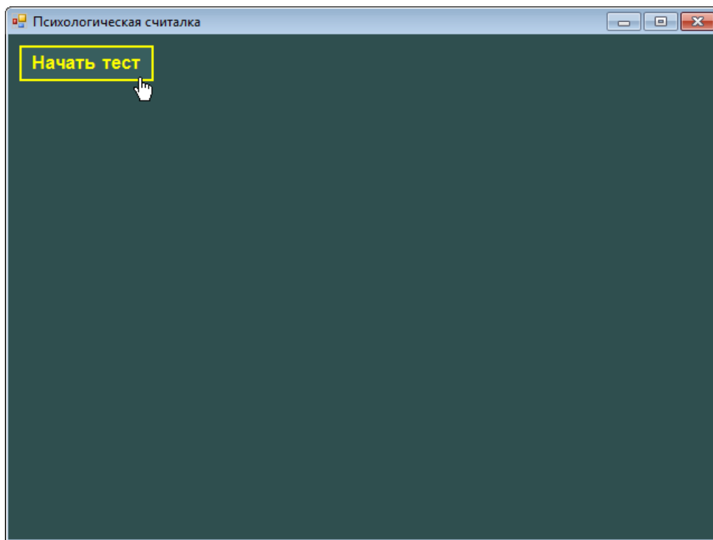
Рис. 34.2. Окно приложения
