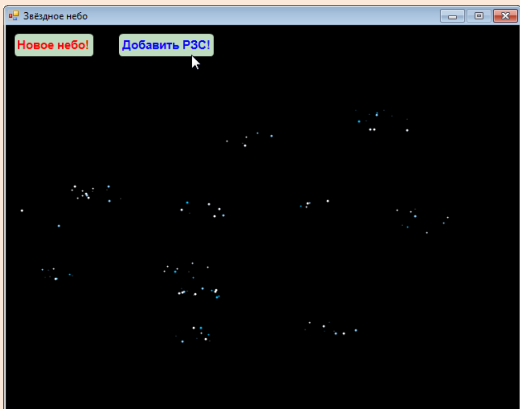
Рис. 35.2. 12 рассеянных скоплений
