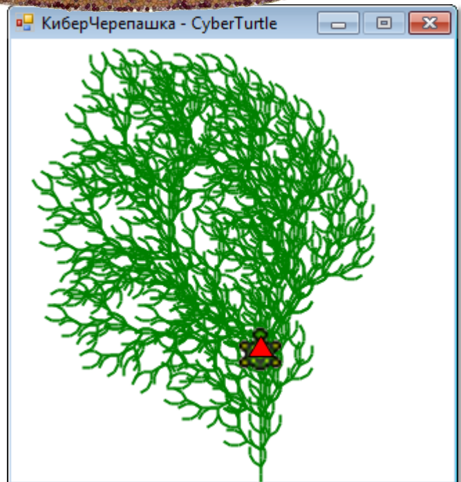
Рис. 23.25. Деревья
