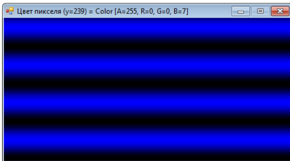
Рис. 19.3. RGB(0, 0, Floor(clr))
