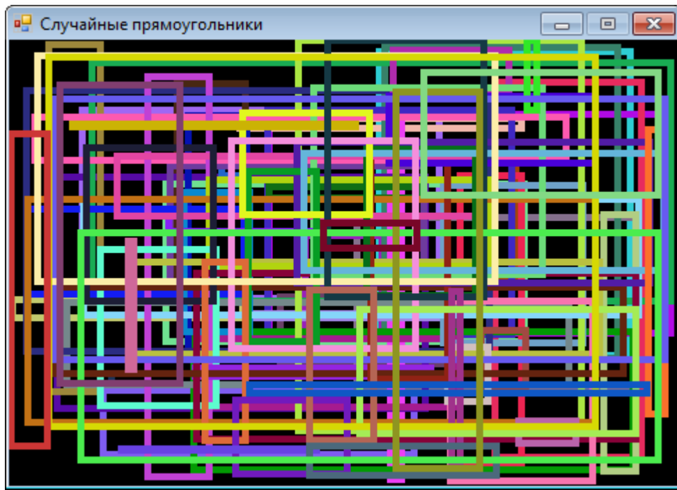
Рис. 21.3. Контурные прямоугольники
