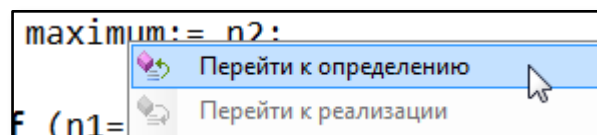
Рис. 9.11. Где начало?
