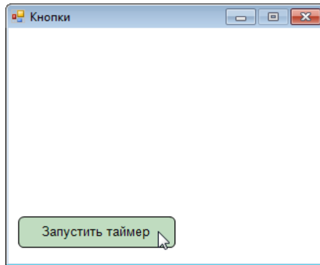
Рис. 25.2. Увеличенная кнопка
