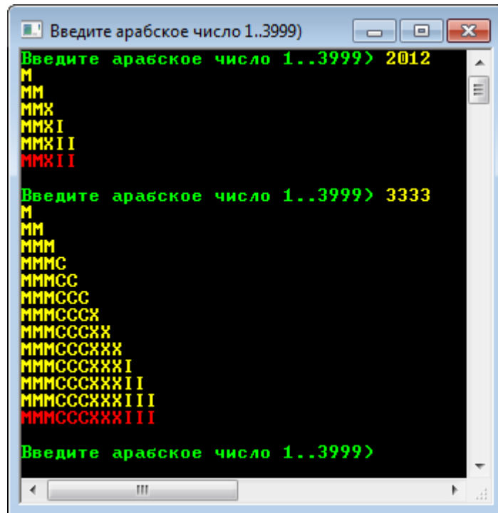
Рис. 7.6. Отладка алгоритма
