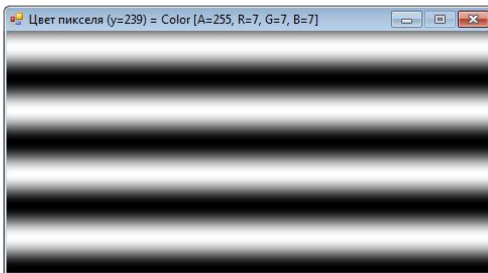
Рис. 19.1. Синусоидные полосы
