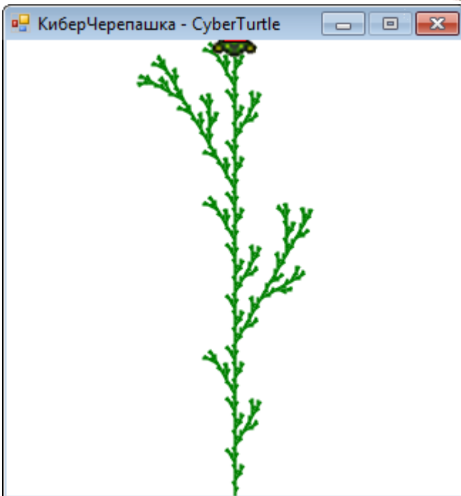
Рис. 23.25. Деревья
