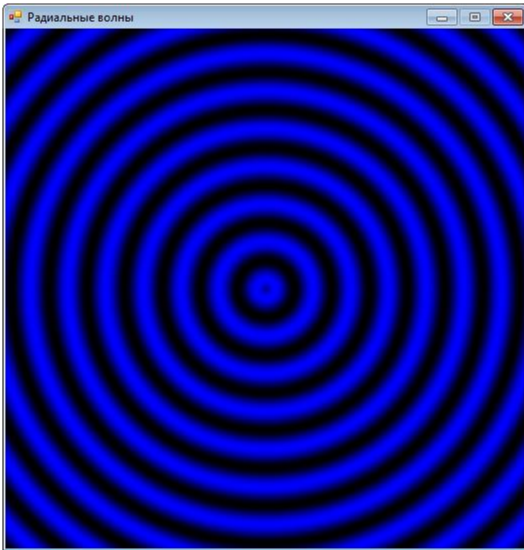
Рис. 19.6. «Полярные» волны!
